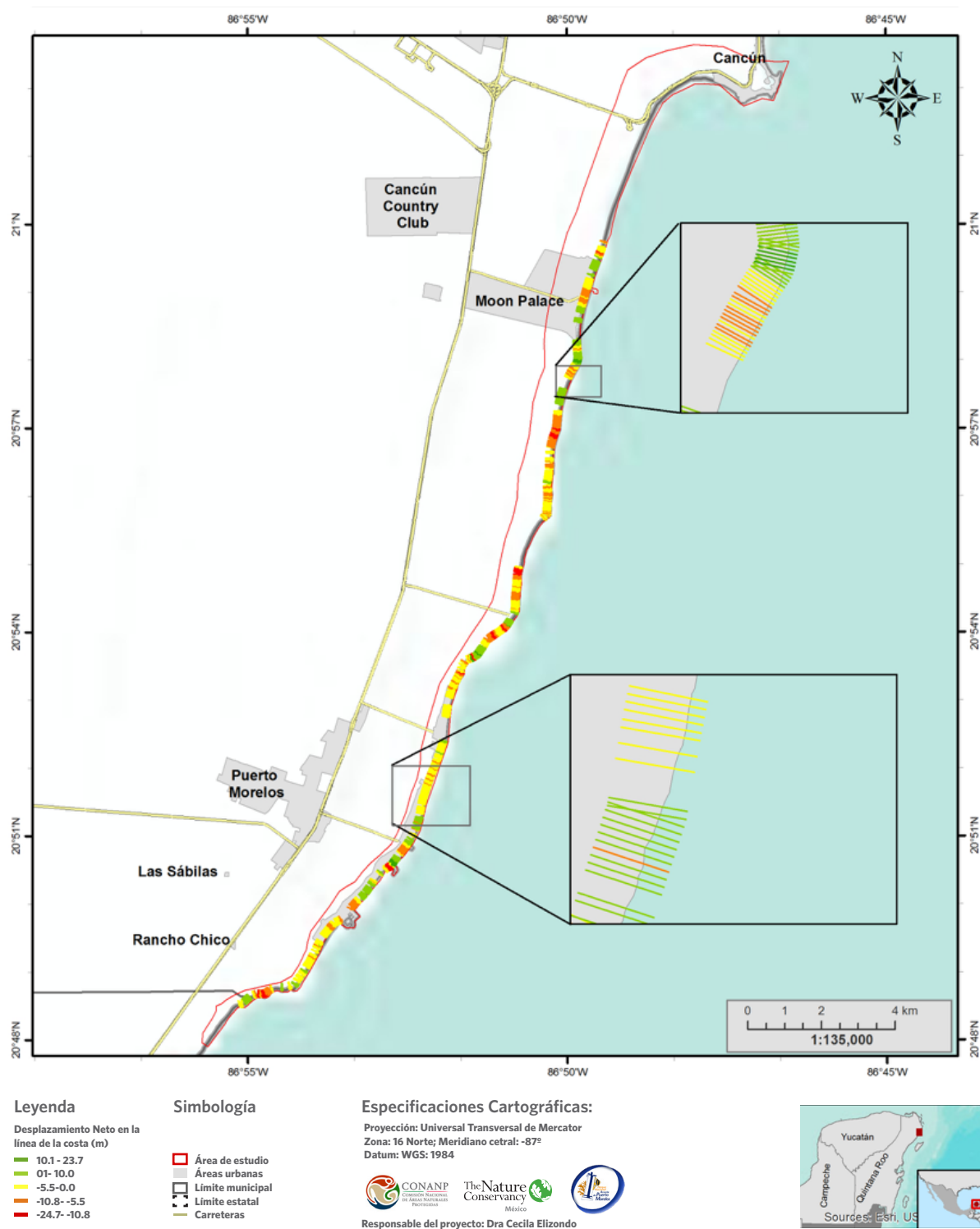
Figura 16: Desplazamiento de la línea de costa entre 2011 al 2017 por segmento. Elizondo, C. et al (2017)
