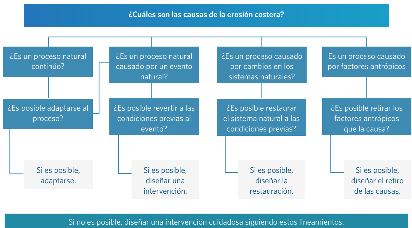
Figura 10: Flujo de preguntas clave para decidir una intervención para el manejo de la erosión.
