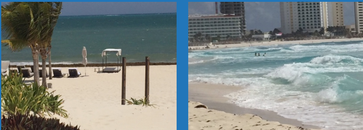
Figura 1: Comparación de la energía del oleaje entre Puerto Morelos, parte de una bahía arrecifal, y Cancún, zona expuesta a mar abierto.
