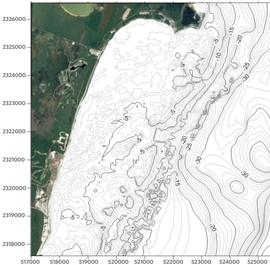
Figura 3: Batimetría de la zona costera de al sur Punta Nizuc, Cancún, Quintana Roo.
