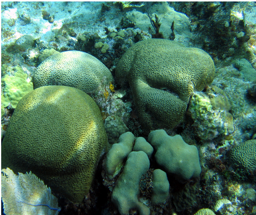
Figura 4: Corales productos de arena.
