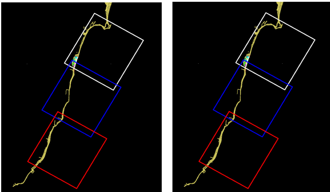
Figura 13: Mallas para utilizar el modelo WAPO y poder abarcar toda el área de estudio de la zona Punta Nizuc - Puerto Morelos.
