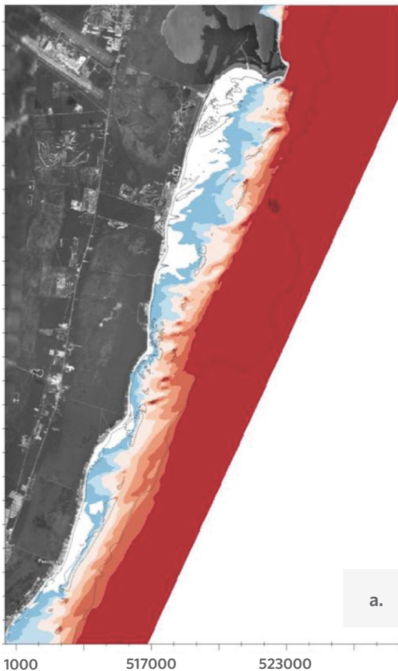
Figura 7: Modelación de la altura de ola significativa por el efecto de la cresta arrecifal del Parque Nacional Arrecifes de Puerto Morelos y Punta Nizuc
